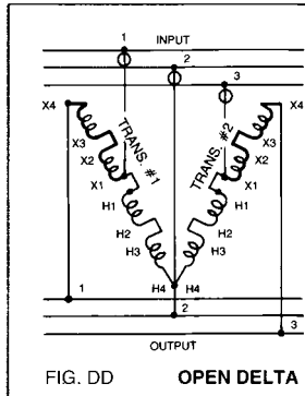
FIG. DD OPEN DELTA
